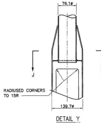
DETAIL Y
