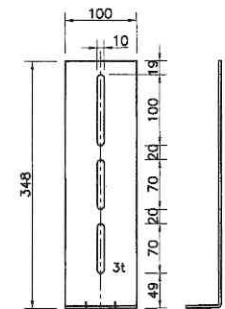
DETAIL Y
