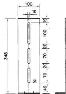
DETAIL Y
